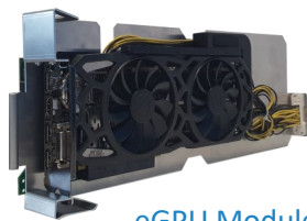
eGPU Module
